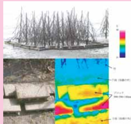
夏に5℃下がる!
