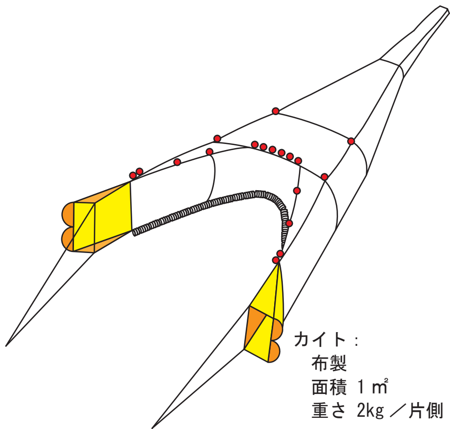
カイト式小型底びき網
