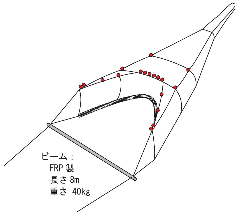
ビーム式小型底びき網（現用）
