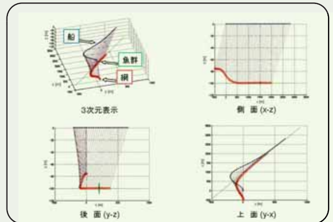
中層トロール漁具 3次元制御
