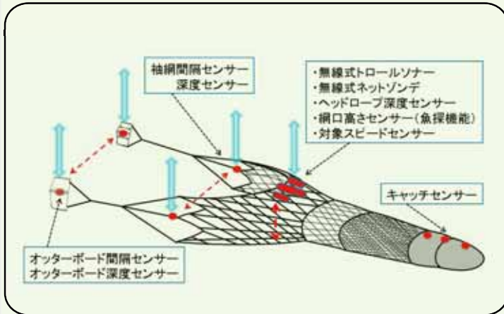
漁具形状測定機の概要
