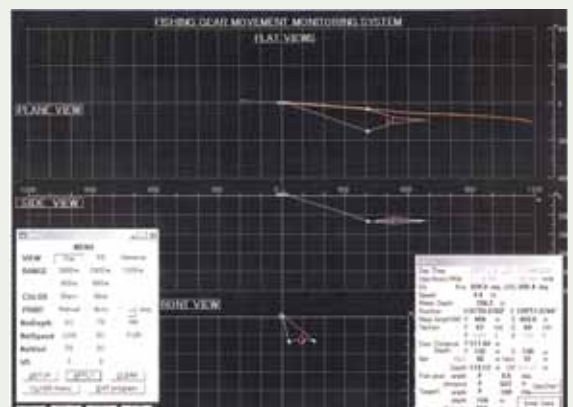
漁具動態監視装置(中層曳き)
