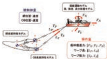
次世代型漁業練習船によるトロール操縦中の制御モデル
